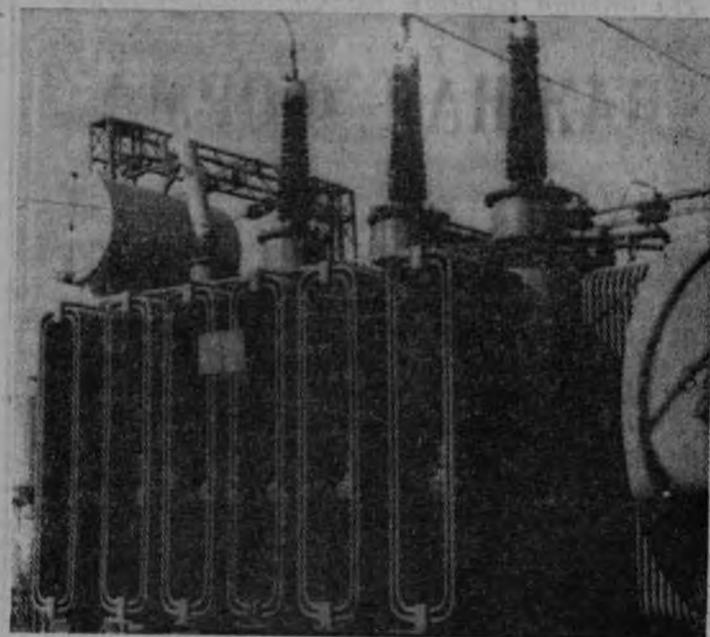
БУГУРУСЛАНСКАЯ ТЯГОВАЯ ПОДСТАНЦИЯ. Здесь смонтирован и действует трансформатор мощностью 31500 киловольт-ампер. Вы видите его на снимке.
