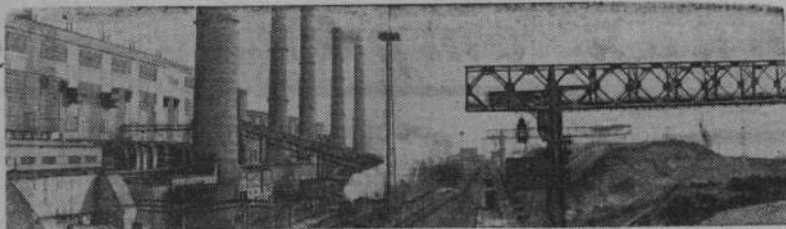
Днепропетровская область. Строители крупнейшей в Европе Приднепровской ГРЭС накануне новой трудовой победы. Закончен монтаж еще одного — тринадцатого — энергоблока мощностью 300 тысяч киловатт. Агрегат вступает в эксплуатацию. НА СНИМКЕ: сегодня на Приднепровской ГРЭС. Фото А. Запары. Фотохроника ТАСС.
