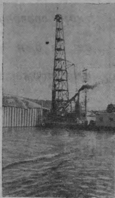
Куйбышевгидрострой. В районе сооружения котлована гидроэлектростанции началась забивка металлического шпунта перемычки, ограждающей котлован. Мощными копрами в дно Волги будет забито свыше 11 тысяч тонн шпунта.
