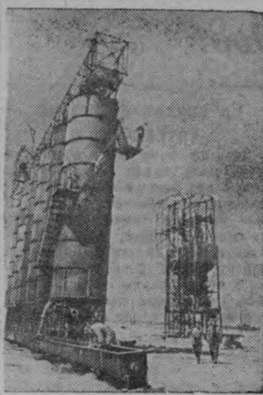
Украинская ССР. На строительной площадке Каховского гидроузла развернуто строительство подсобных предприятий. На 2 м участке строится бетонный завод. НА СНИМКЕ: монтаж бетонного завода на строительной площадке 2 го участка.
