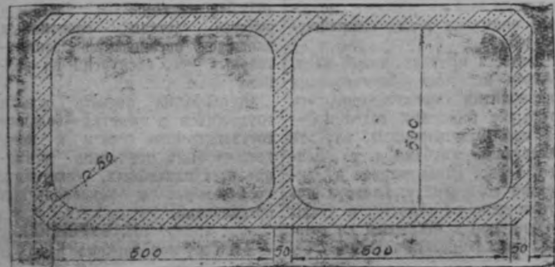
План траншеи на 200 тонн силоса с одной перемычкой.
